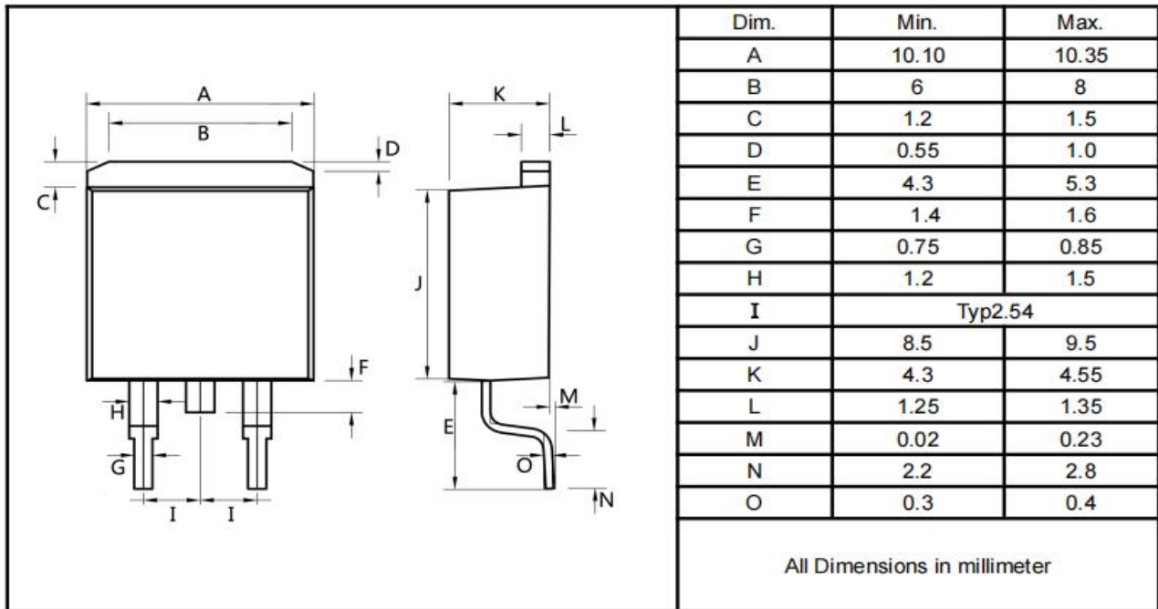
T0-263
